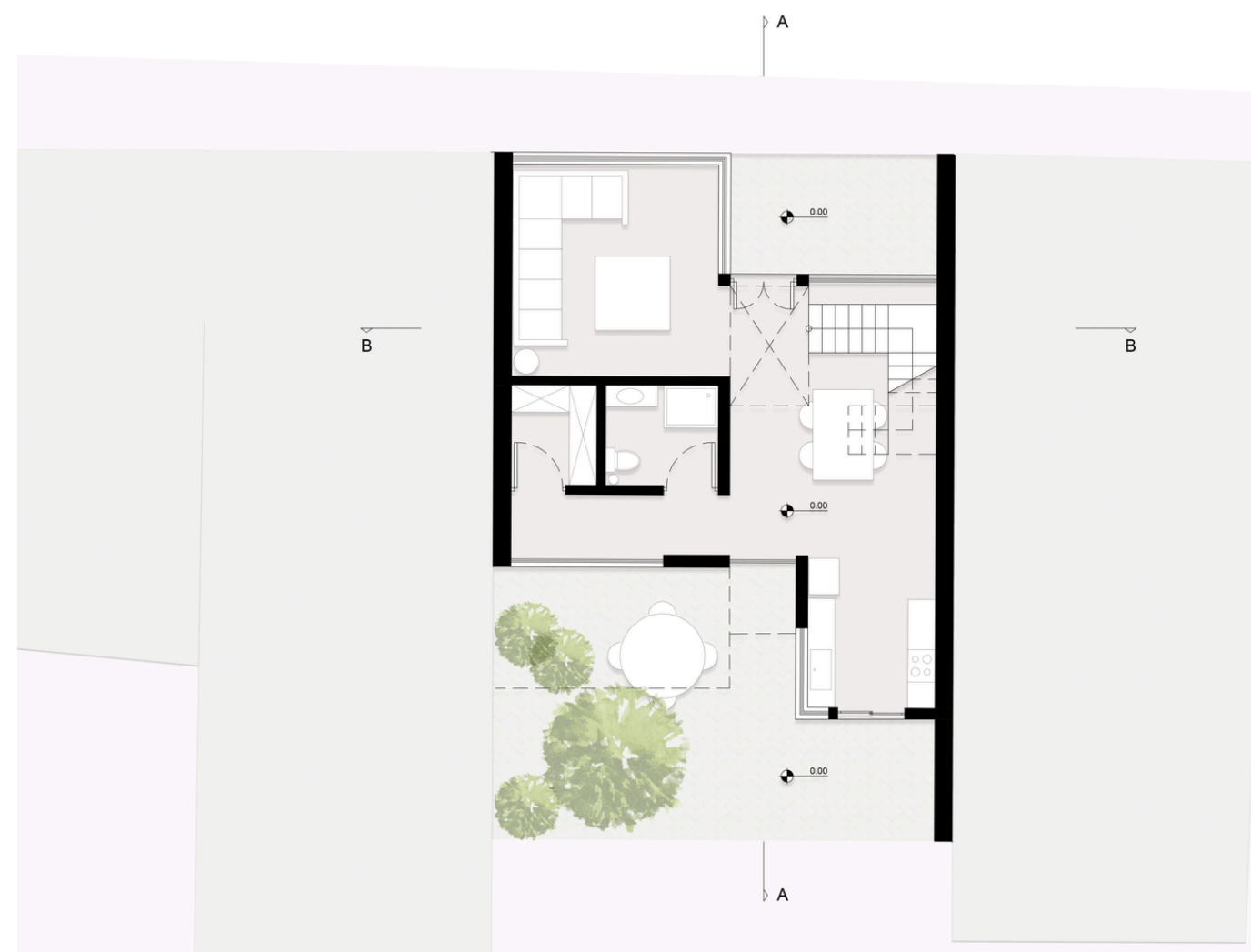
ΚΑΤΟΨΗ ΙΣΟΓΕΙΟΥ
