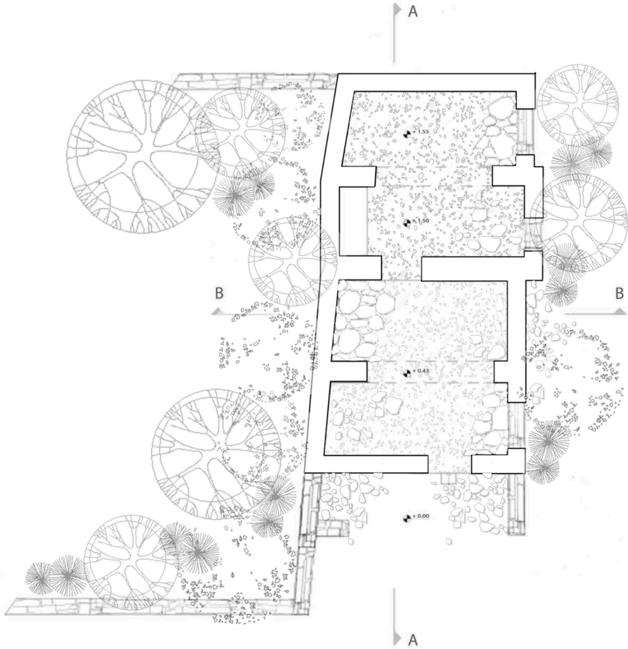
ΑΡΧΙΤΕΚΤΟΝΙΚΗ ΑΠΟΤΥΠΩΣΗ ΚΑΤΟΨΗΣ
